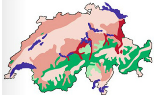
1. Windlastkarte nach SIA 261
